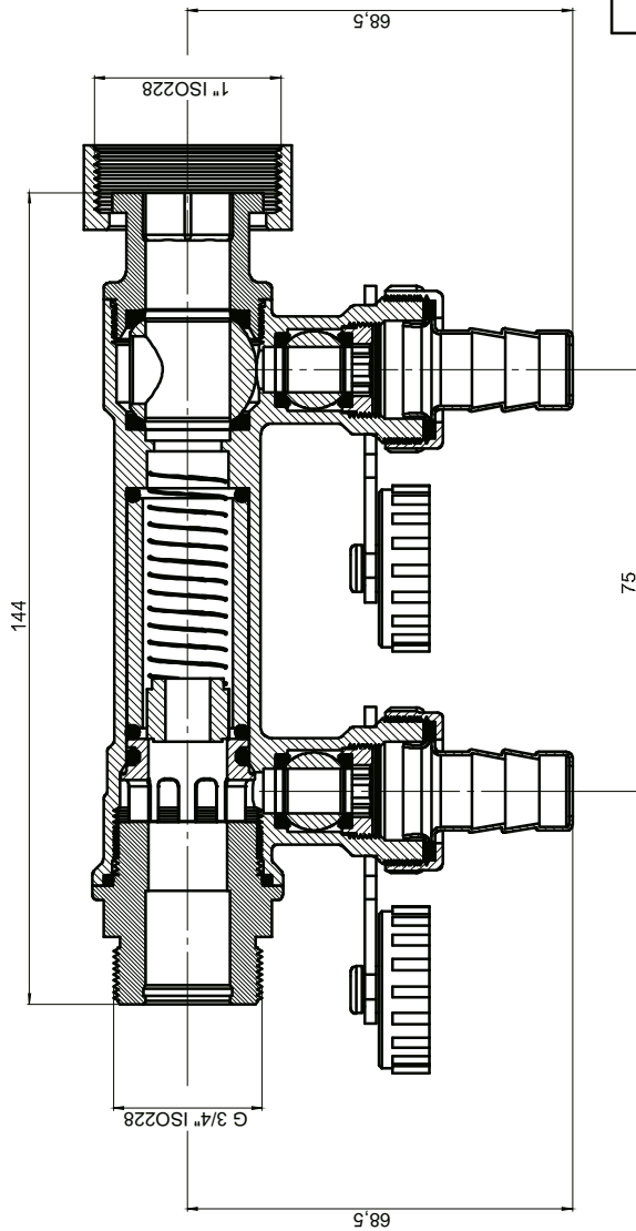
SEZIONE A-A
