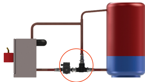
Laddomat 11 wird zwischen Kessel und Pufferspeicher platziert
