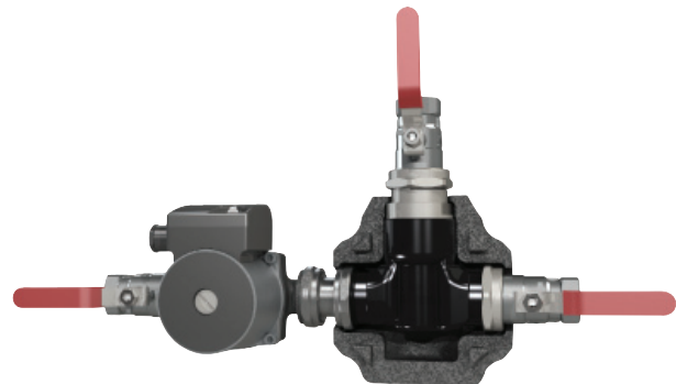
Laddomat 11-200
